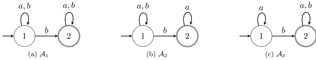
FIGURE 1 – Trois automates reconnaissant le même langage
